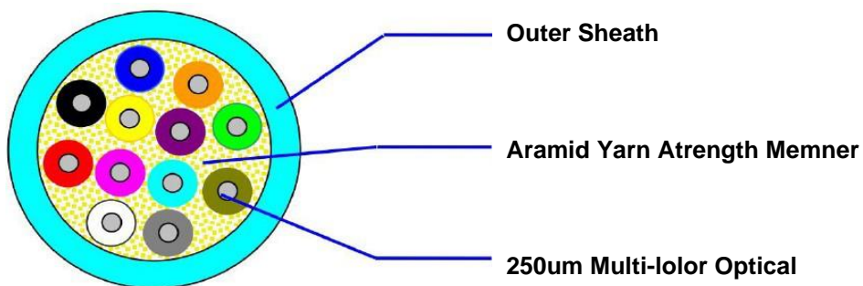
MIC: 250um mini round cable
